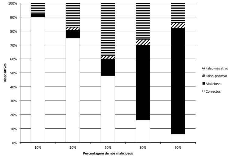
Figura 7. Robustez a dispositivos maliciosos
